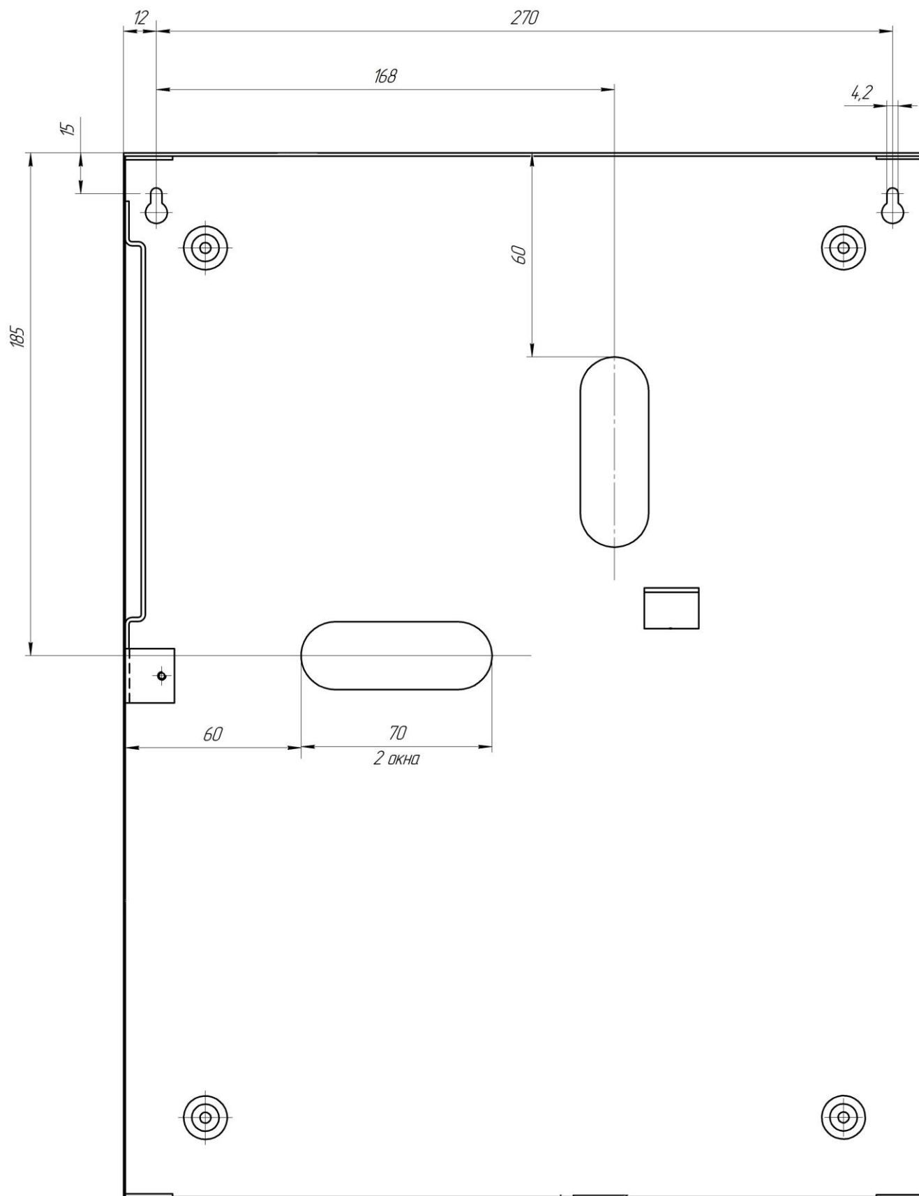
Рисунок Е.1 – Розмітка отворів кріплення базового блоку
