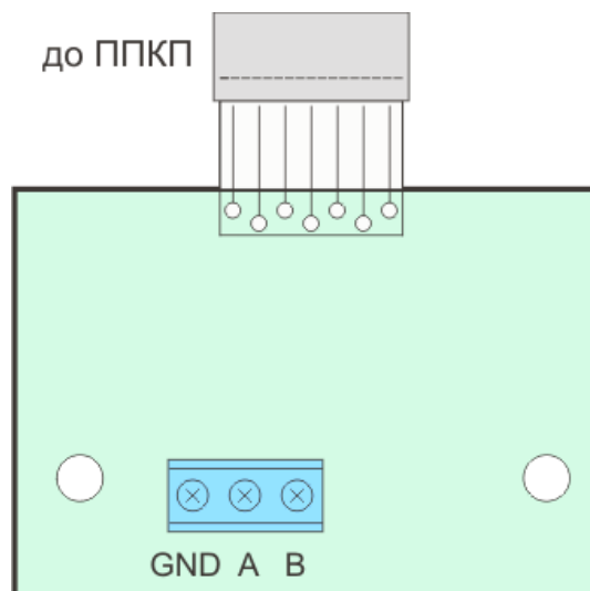
Рисунок 7.6 – Модуль МКІ
