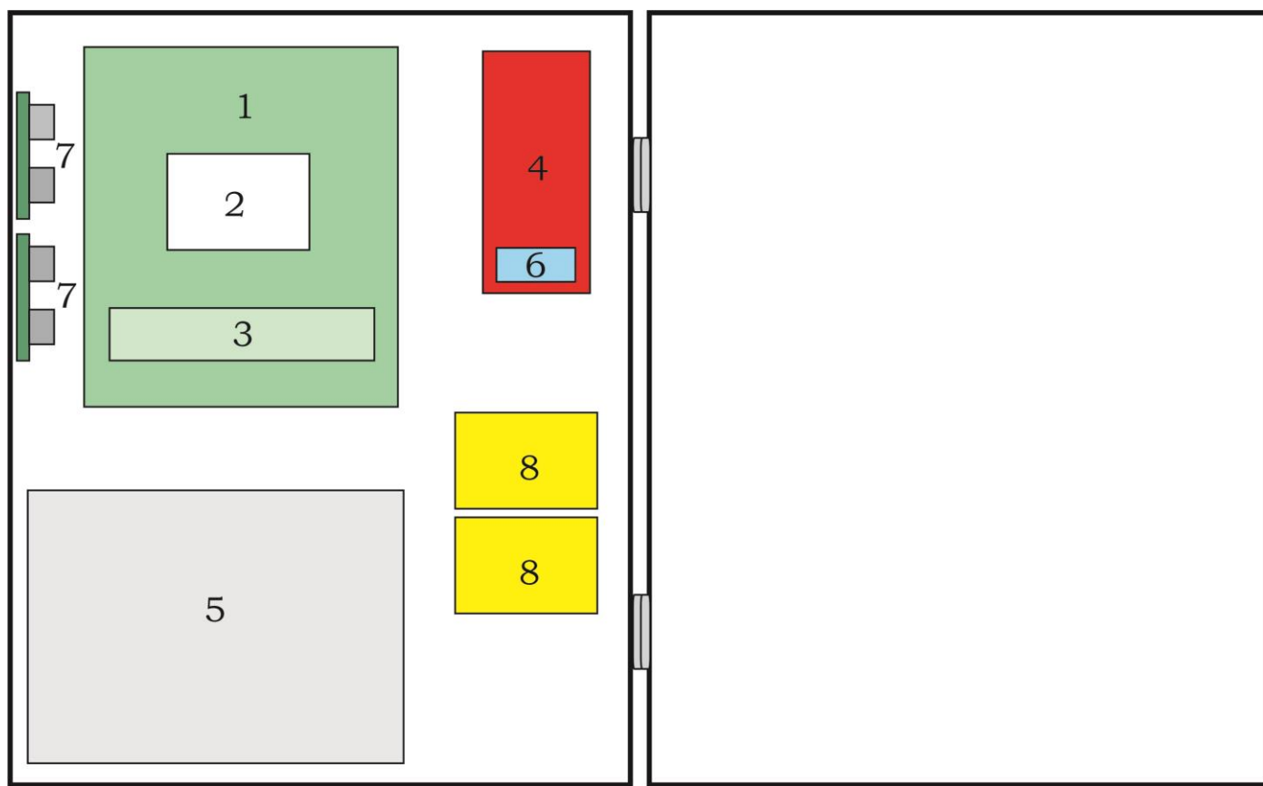
Рисунок Г.1 – Розміщення блоків та модулів в корпусі приладу
