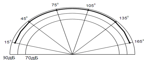
Мал. 2 Акустична діаграма показника
