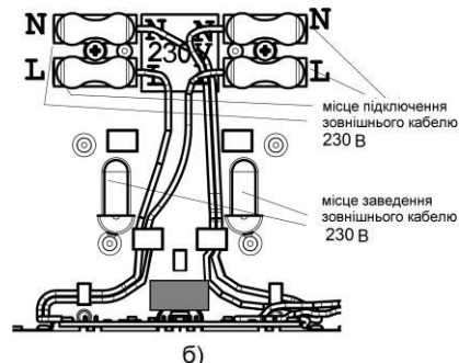
Мал.3 Підключення кабелю живлення для виконань:
