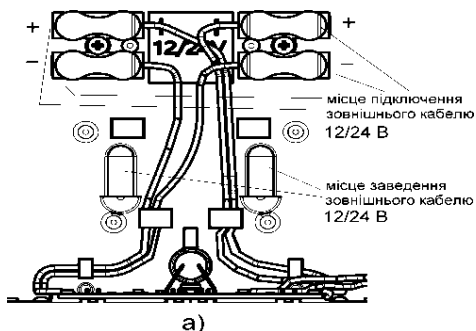
Мал.3 Підключення кабелю живлення для виконань:
